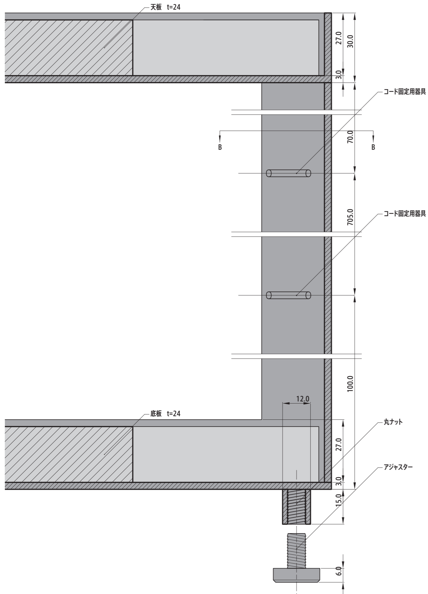
SECTION A-A
